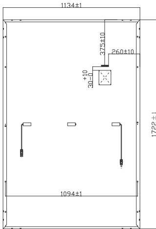
背面図
