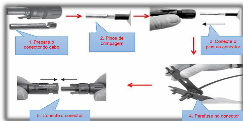
Figura 23. Método de produção do conector de cabo
