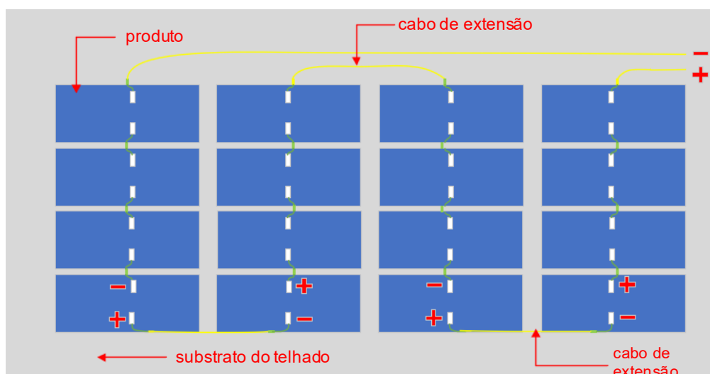
Figura 22. Instruções de operação da conexão do jumper do produto (vista frontal)
